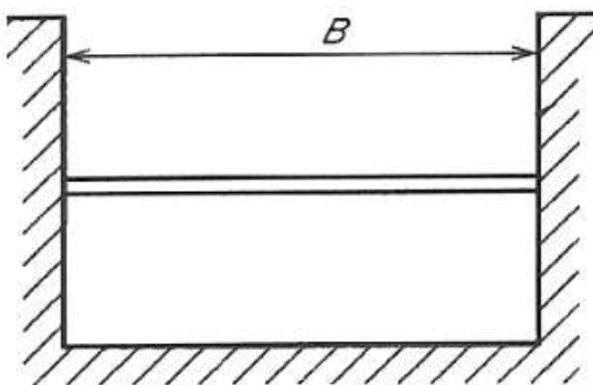
< 전폭 위어 >
